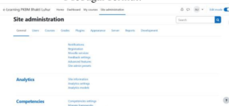
Gambar 12. Administrasi Situs
